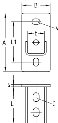
MPC-nyeregalakú rögzítő, hosszirányú
