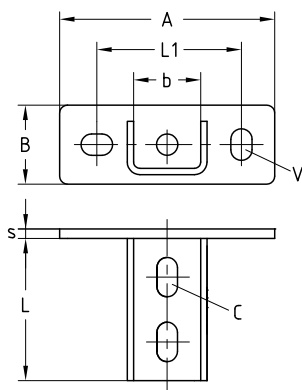
MPC-nyeregalakú rögzítő, keresztirányú
