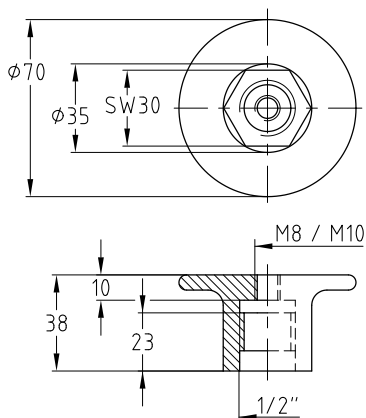
Fixpont szerelés csőmenetcsatlakozású csavaros csőbilincssel
