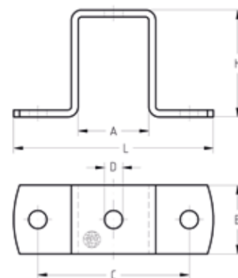
40/60 profilhoz
