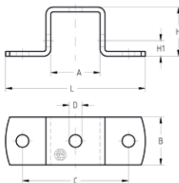
28/30 és 38/40 profilhoz
