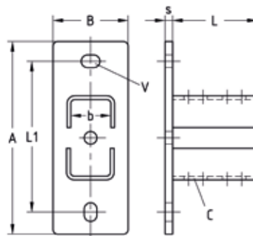
MPC-nyeregalakú rögzítő, hosszirányú 38/80, 40/80 és 40/120 profilhoz
